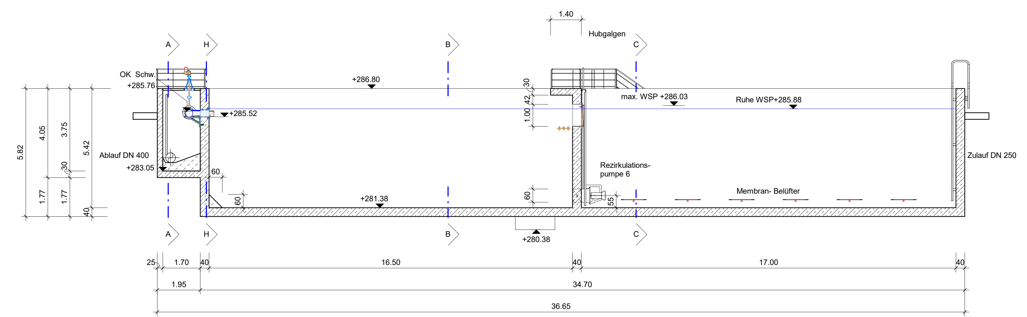
Schnitt E - E
