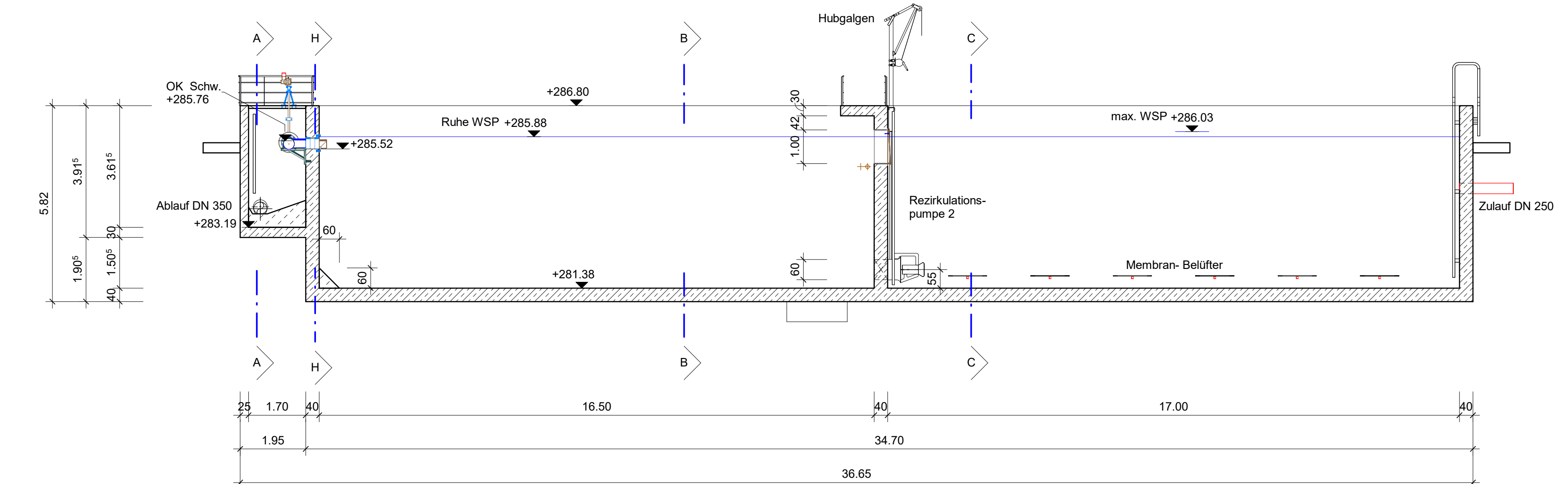
Schnitt F - F
