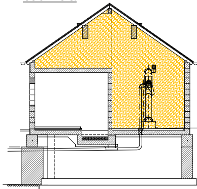
COUPE C-C.
