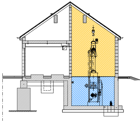
COUPE A-A.
