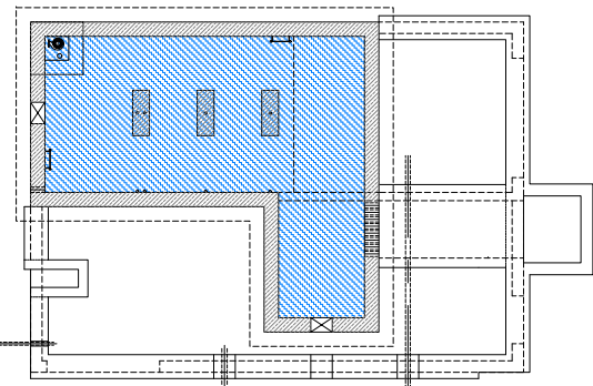
VUE EN PLAN - CAVE
