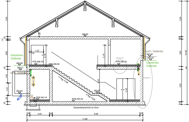
Schnitt B-B
