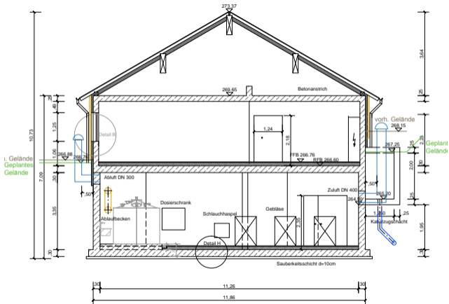
Schnitt C-C
