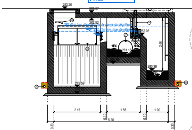
COUPE E-E
