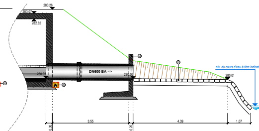
COUPE J-J
