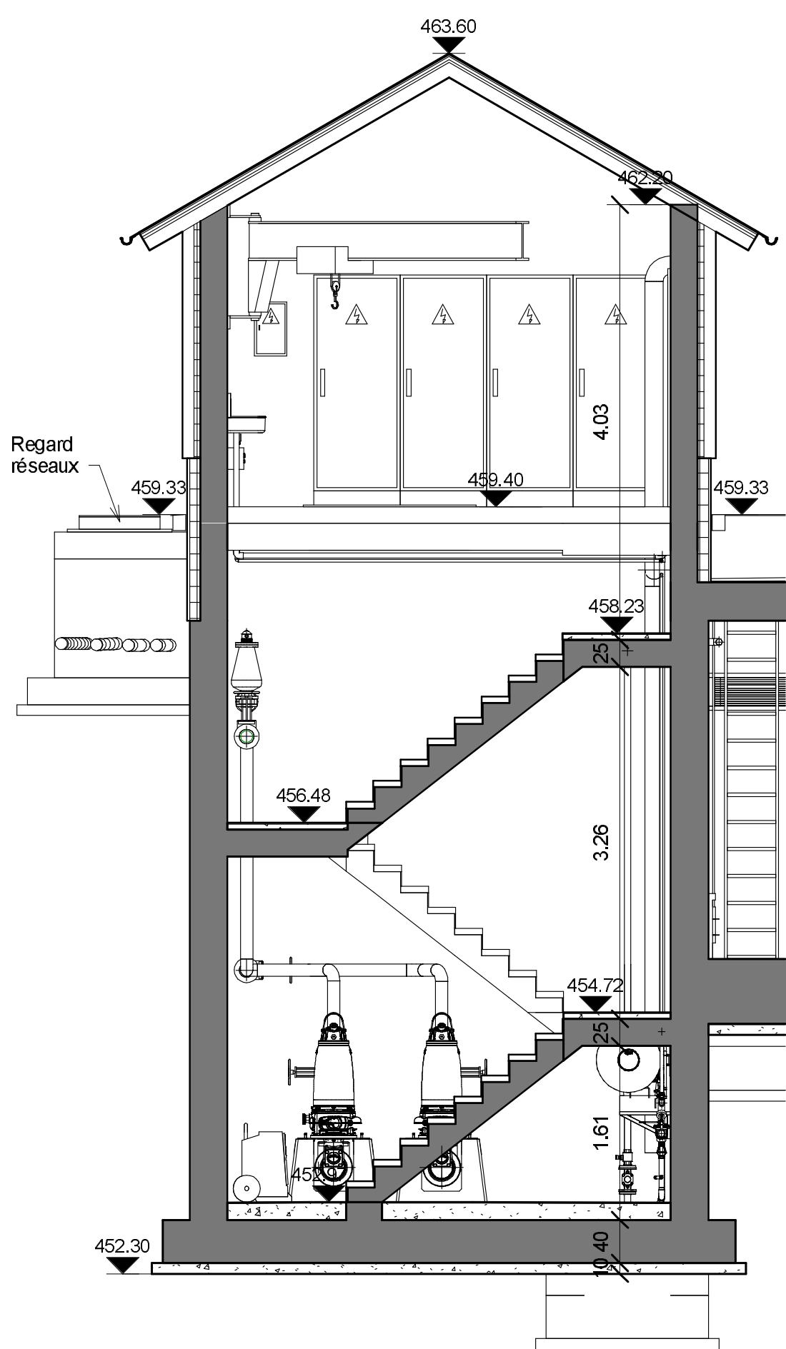
Coupe EE
