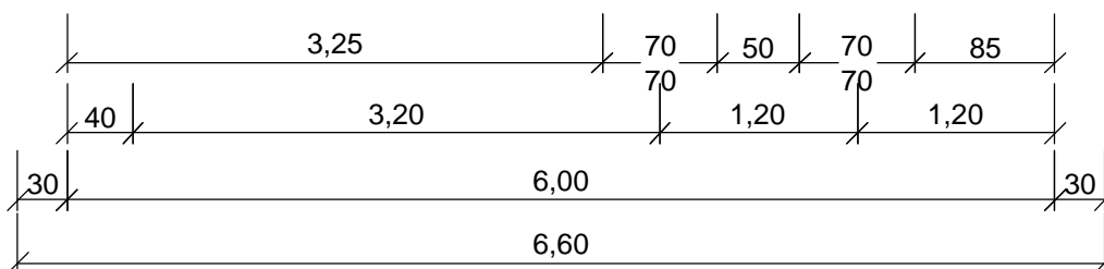
SCHNITT E-E
