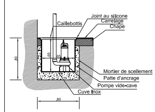
Détail puisard (1:20)
