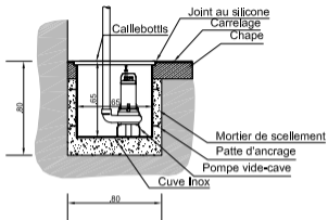
Détail puisard (1:20)
