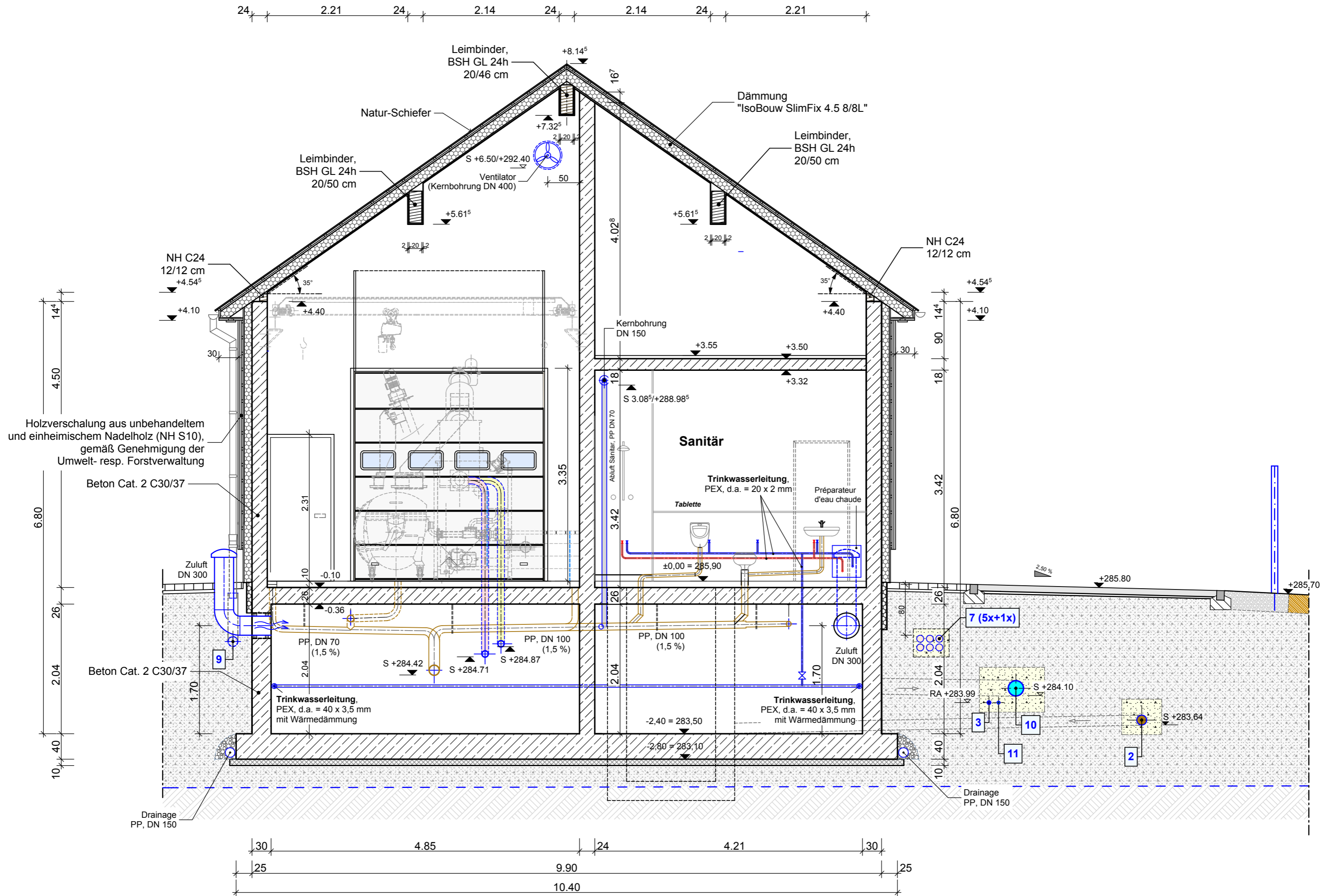
Schnitt 1 - 1
