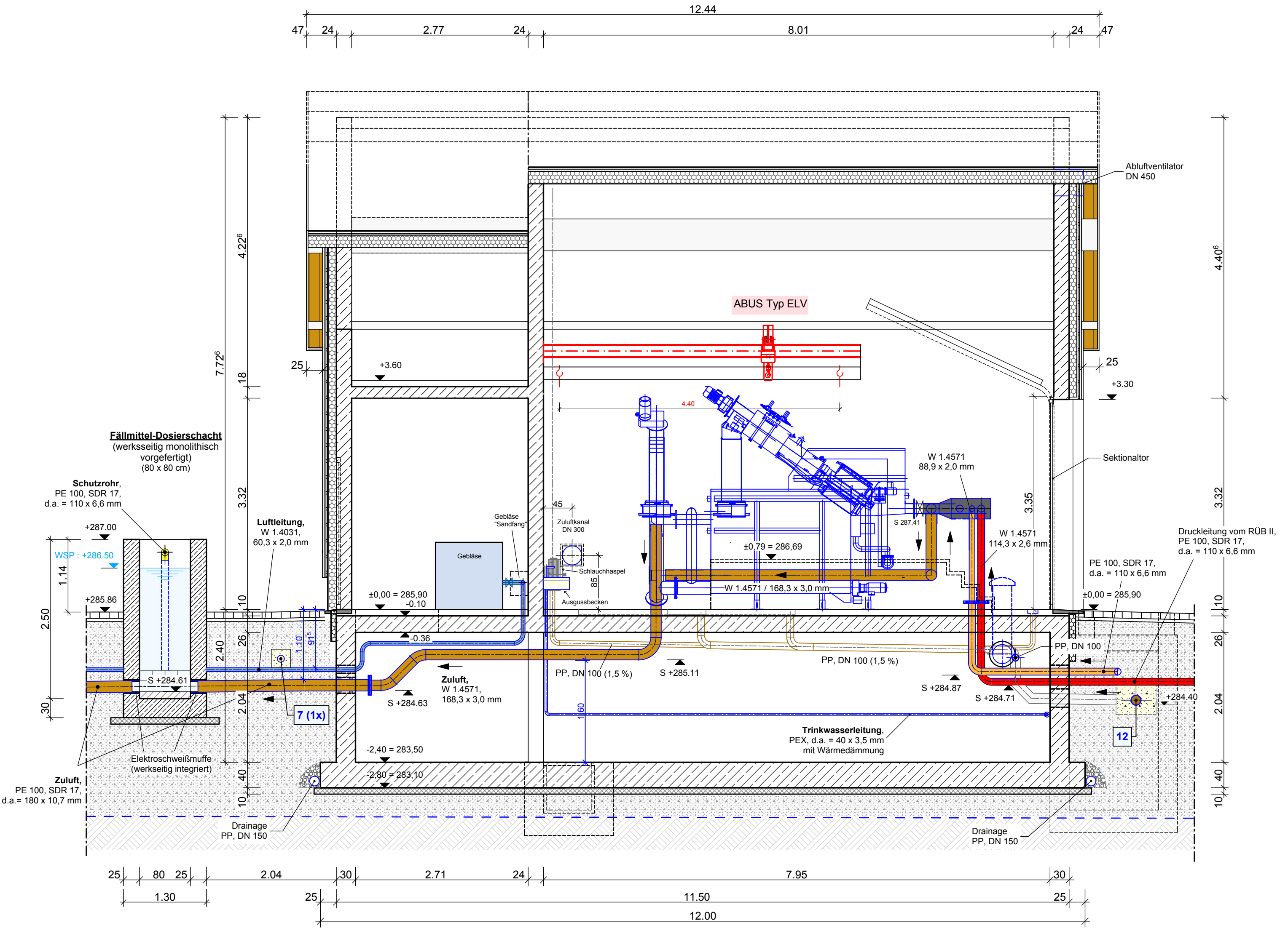
Schnitt 4 - 4
