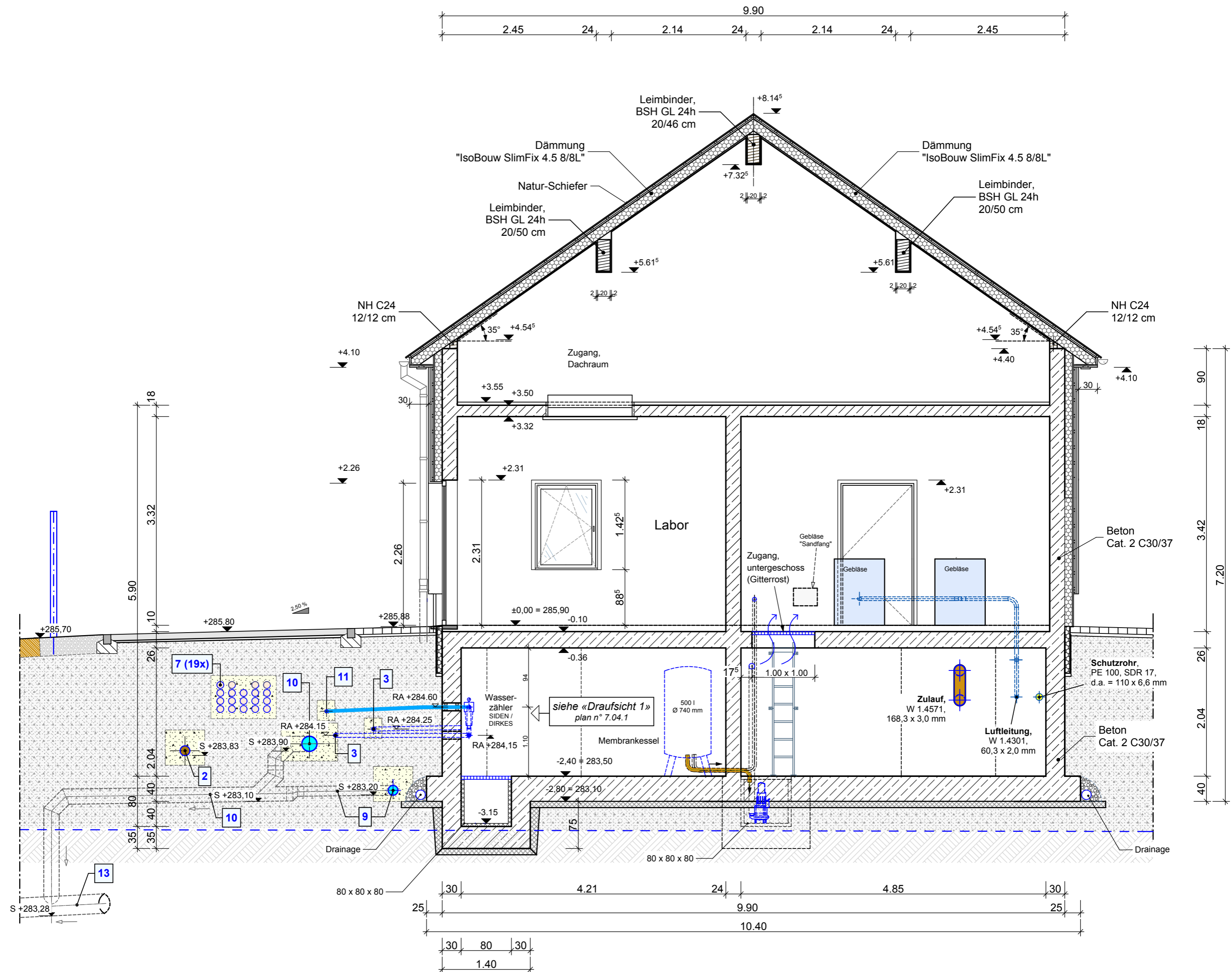
Schnitt 3 - 3
