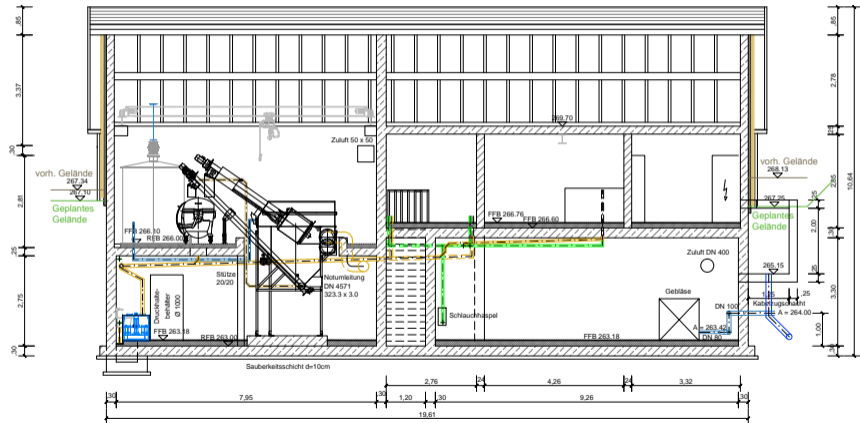
Schnitt D-D
