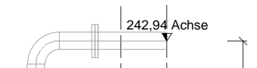
Detail Ausbildung Saugleitung DN150 Druckleitung DN100 M 1:25
