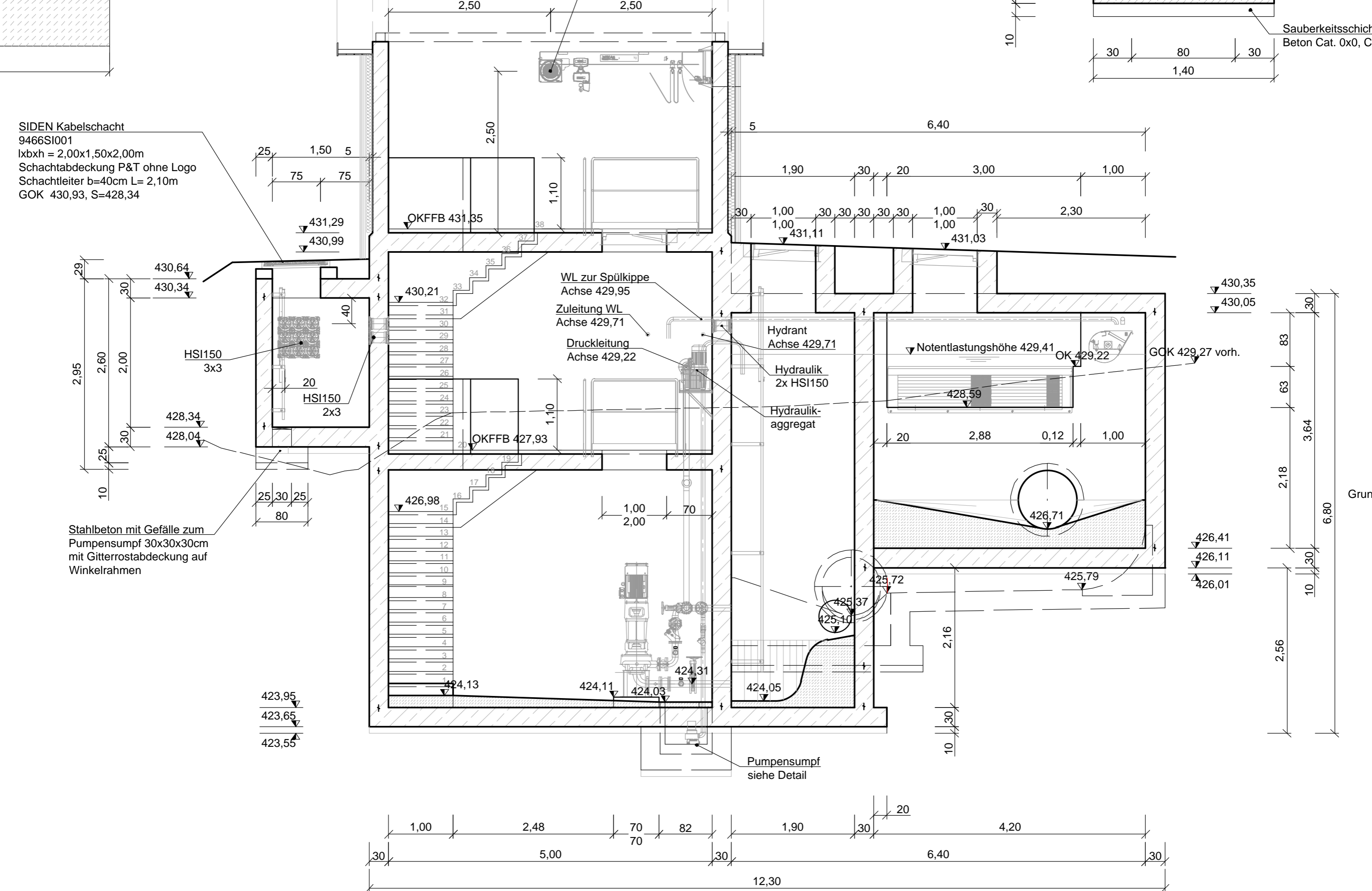
SCHNITT B-B
