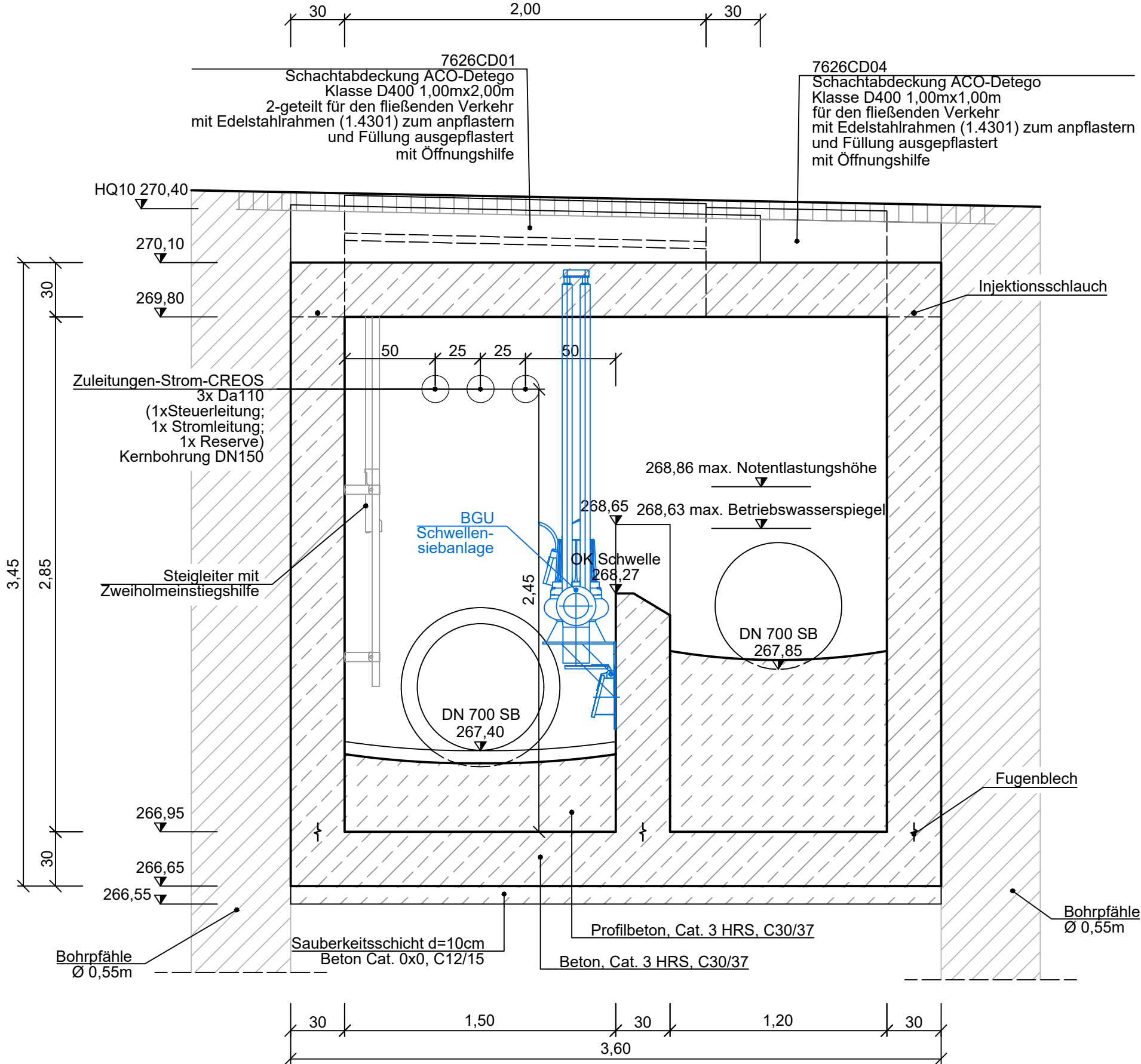
SCHNITT C-C
